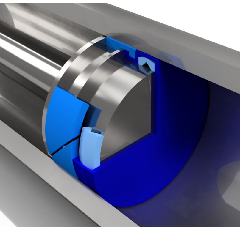
Guarnizione composta fornita in KIT: tenuta frontale + fascia di guida
