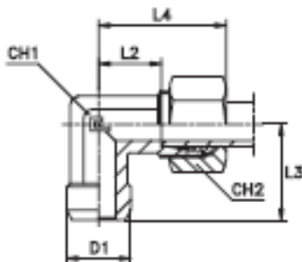
Tipo: 1058.. Anello B3
