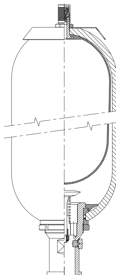
Attacco fluido SAE 3000 e 6000
